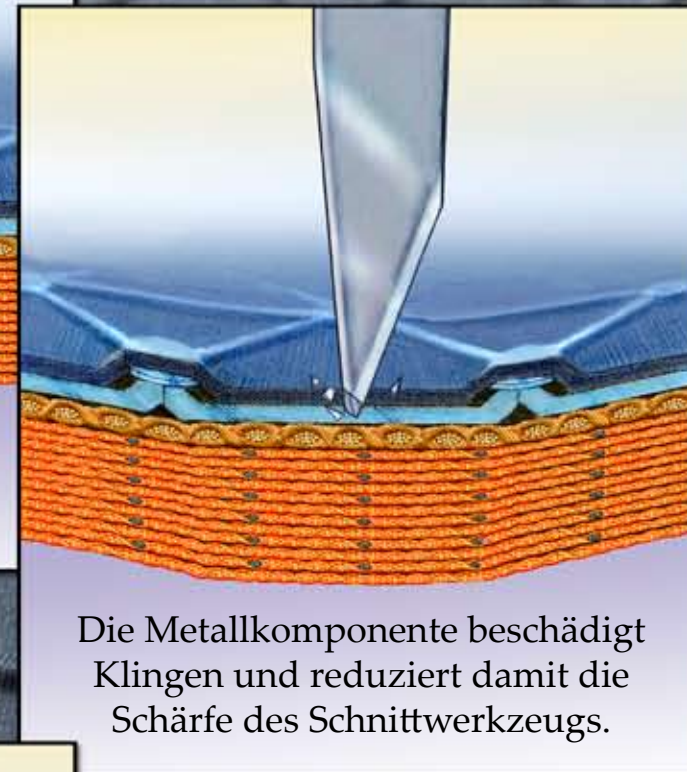
Das flexible MFA-Schichtsystem
