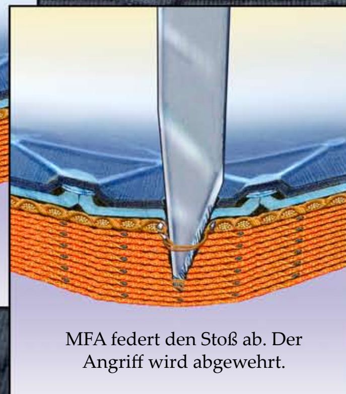
Die TurtleSkin-Schicht fängt die Klinge ab.
